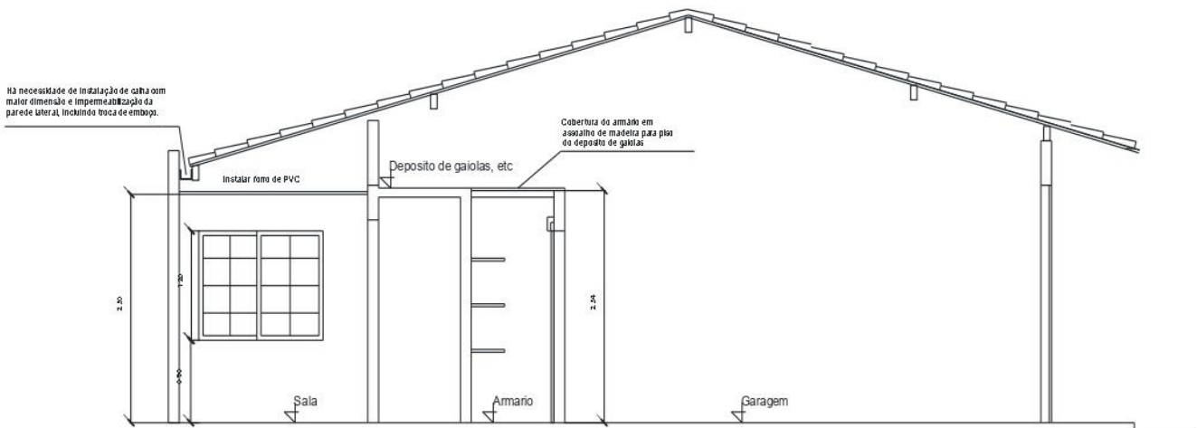
Corte esquemático AB
