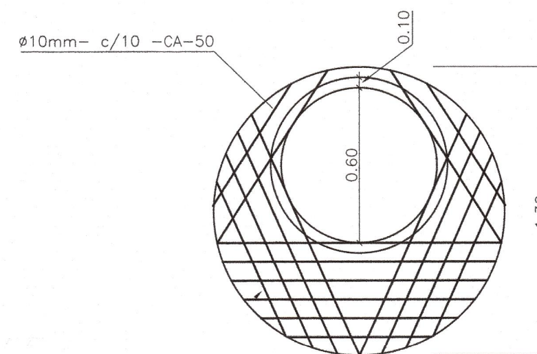
PLANTA DA LAJE CAPOEIRA
