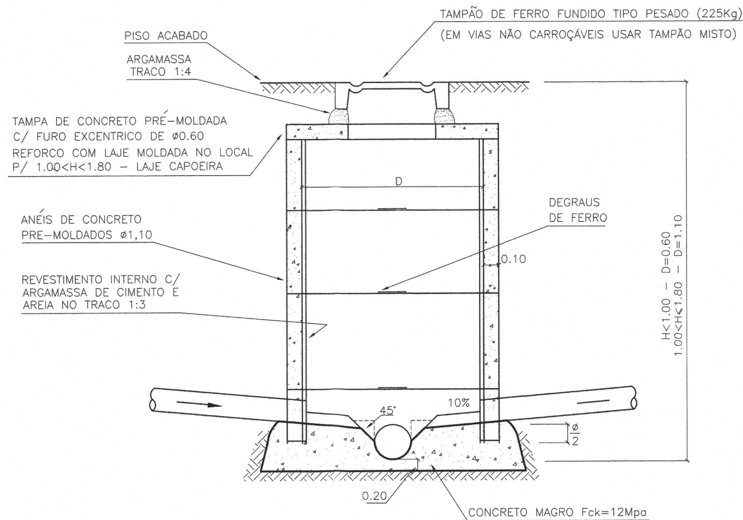
CORTE B-B
